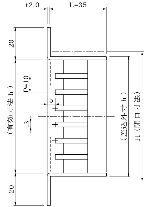
B-B 断面図
