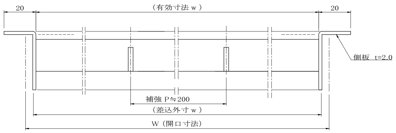
A-A 断面図
