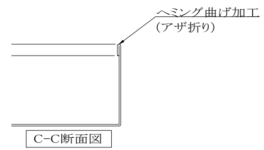
D部詳細図
